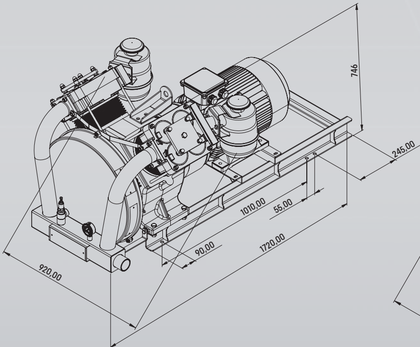
► G220-2 ELEKTRİKLI MOTORLU ELECTRICAL ENGINE / С ЭЛЕКТРОДВИГАТЕЛЕМ
