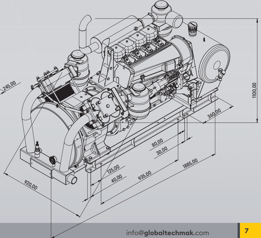
► G220-2 YENİ DİZEL MOTORLU NEW DIESEL ENGINE / С НОВЫМ ДИЗЕЛЬНЫМ ДВИГАТЕЛЕМ
